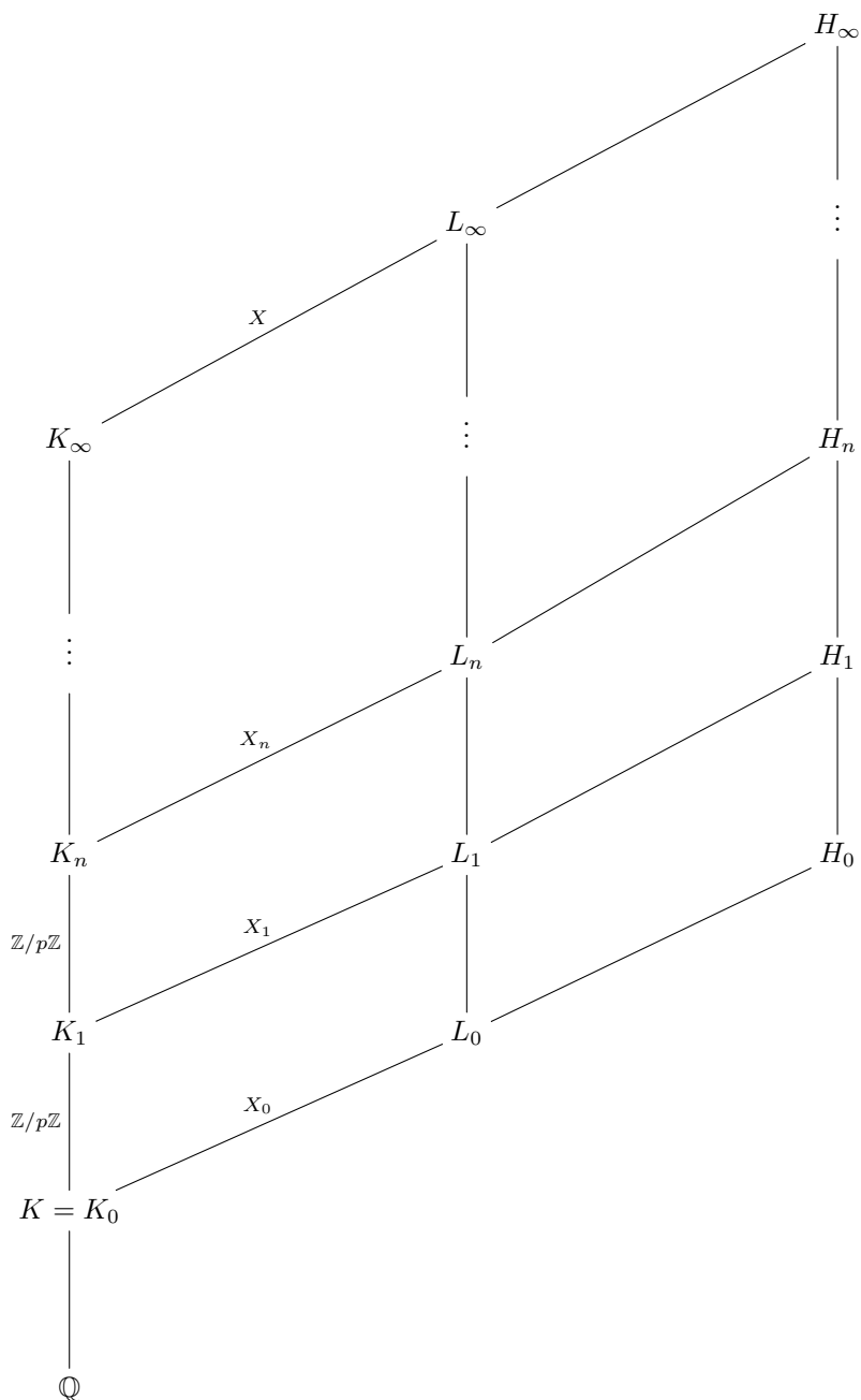
Figura 9: La \mathbb{Z}_p -extensión K_\infty/K , la máxima p -extensión abeliana sin ramificación de la capa K_n , y sus cuerpos de clases de Hilbert.
