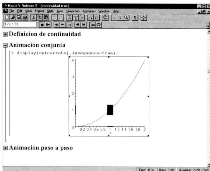
FIGURA. Maple 2
