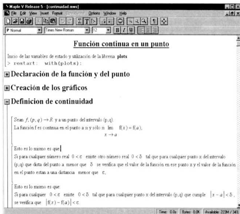
FIGURA. Maple1
